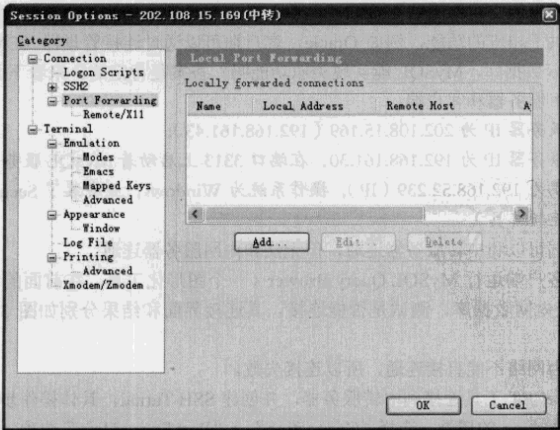
图 31-3 Session Options 设置界面
