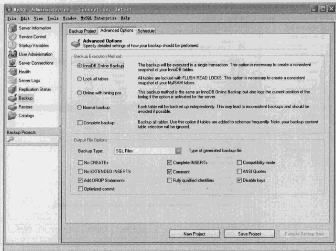
图 6-5 MySQL Administrator 备份管理
