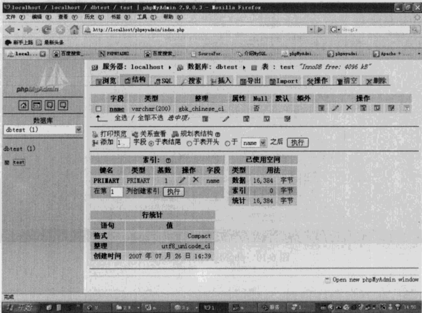
图 6-9 phpMyAdmin 表管理维护页面
