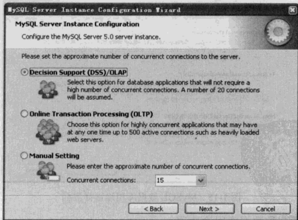
图 1-17 MySQL 并发连接设置界面
