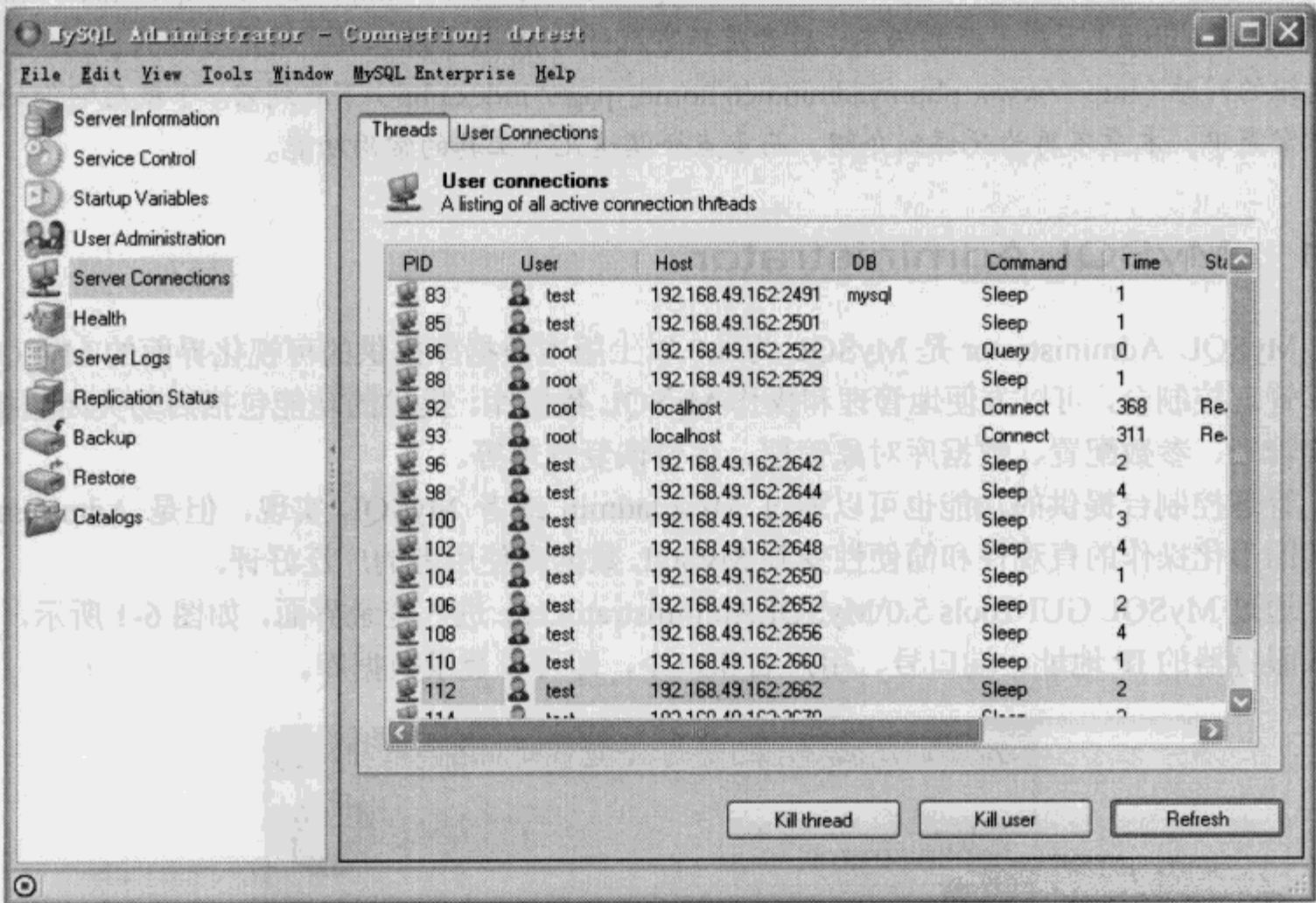
图 6-2 MySQLAdministrator 连接管理
