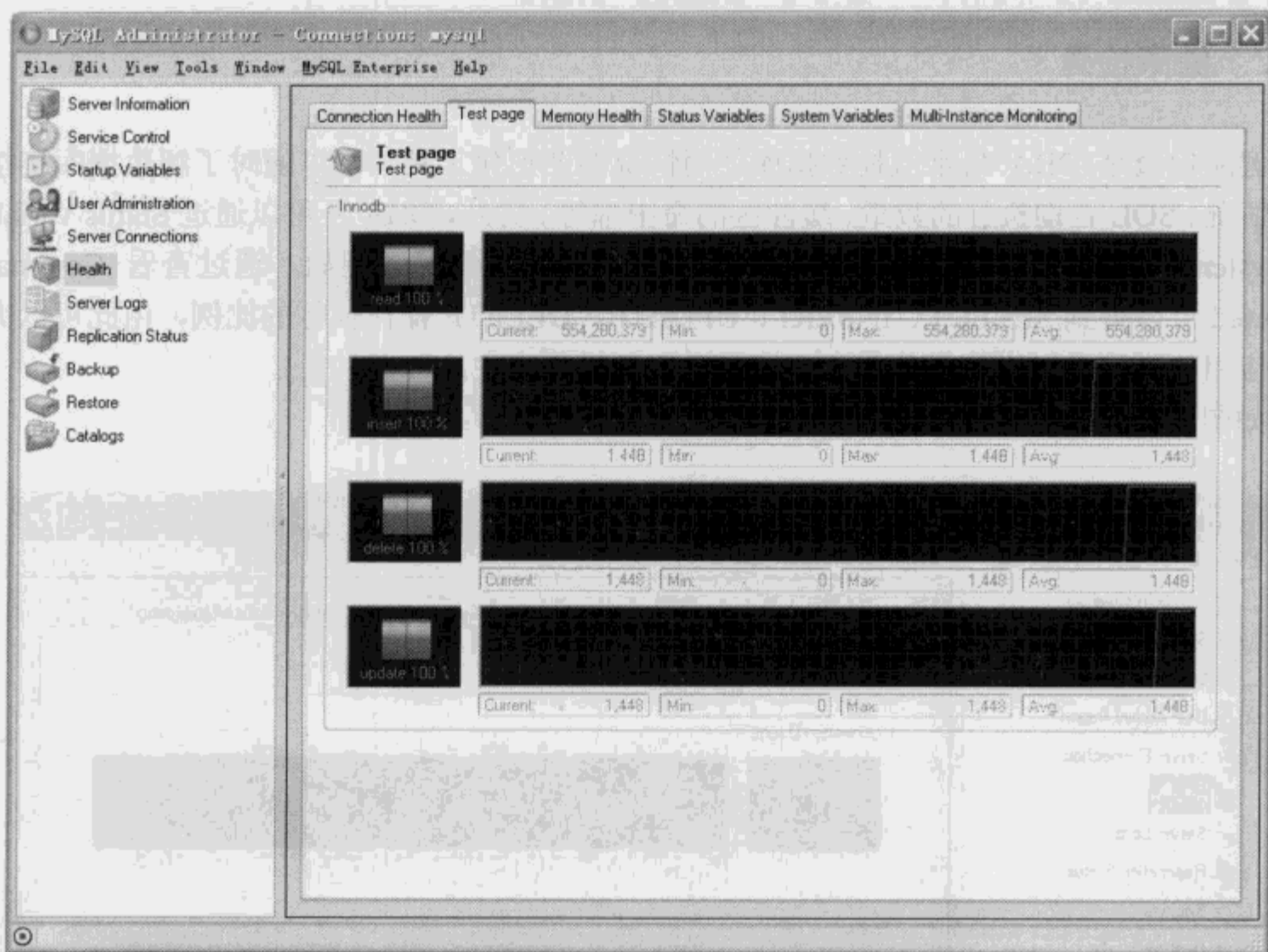
图 6-4 MySQL Administrator 健康检查-自定义监控内容
