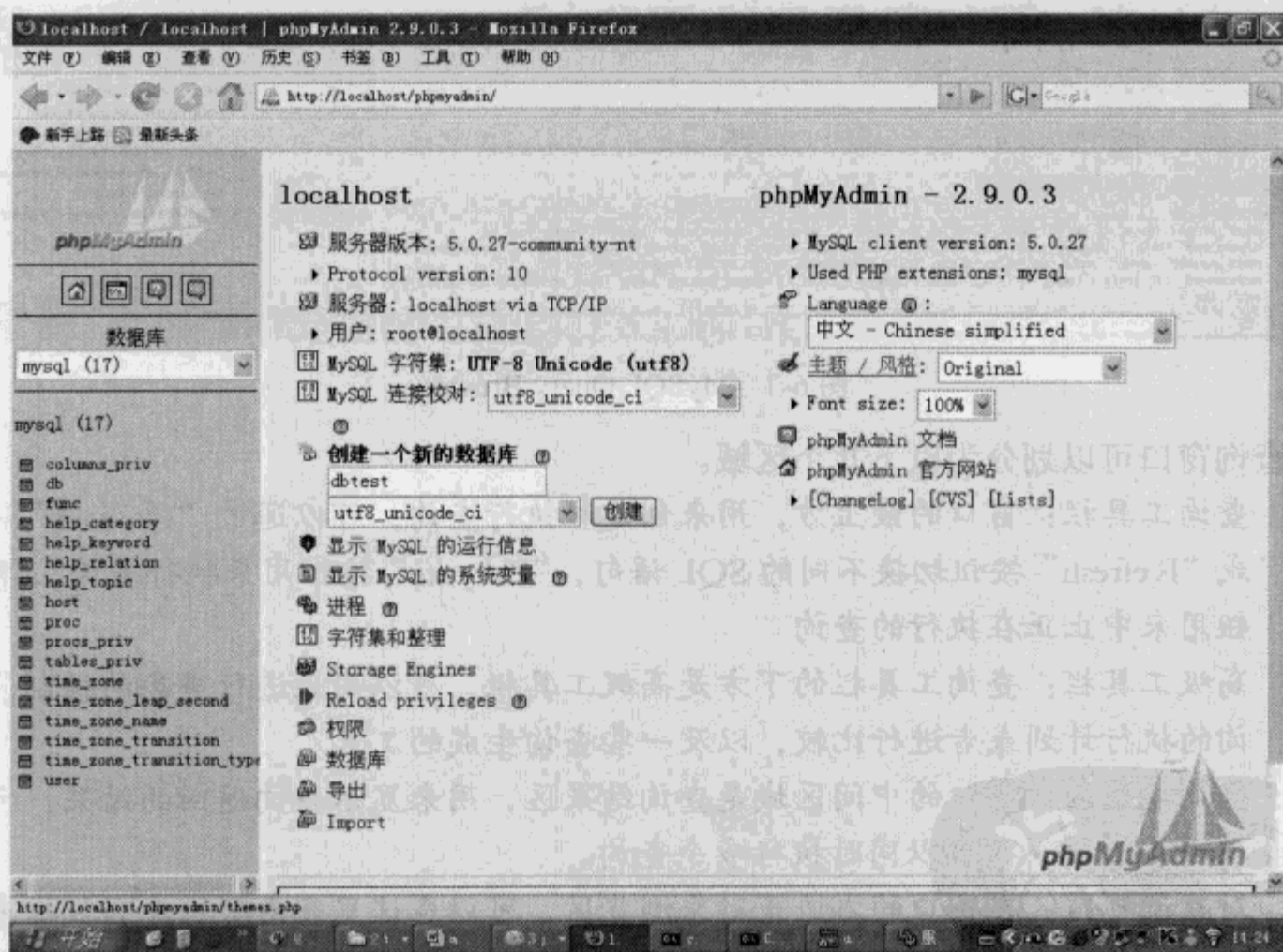
图 6-8 phpMyAdmin 主页面
