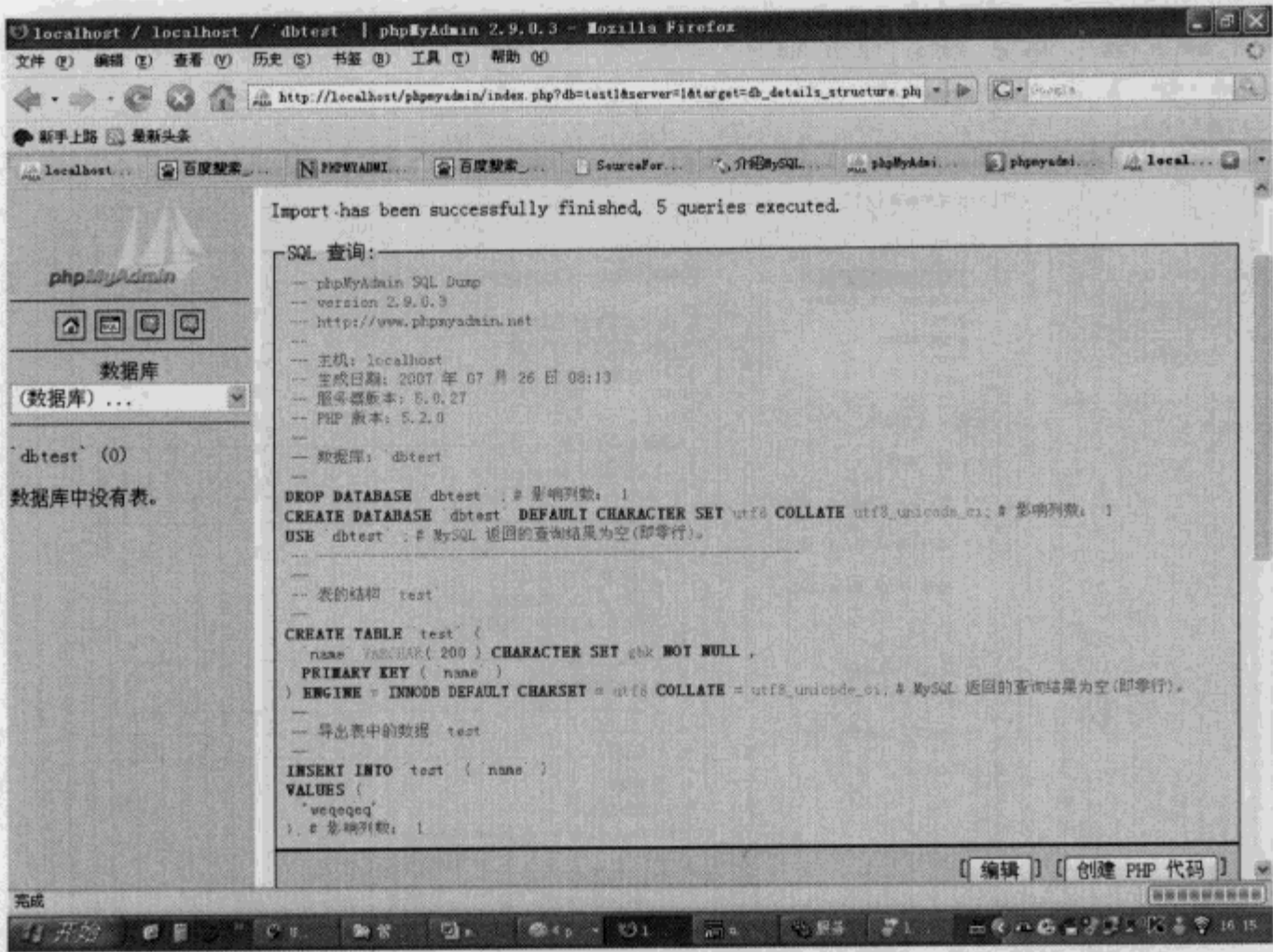
图 6-13 phpMyAdmin 导入成功显示
